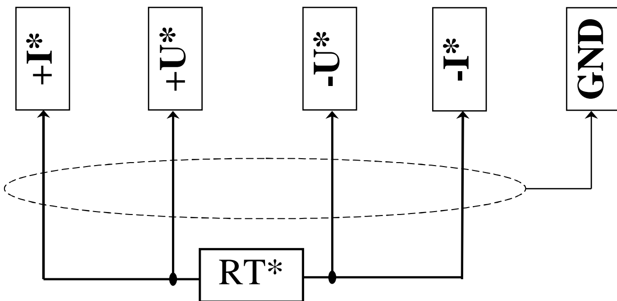
Рисунок Г.2 – Подключение датчиков температуры (по каждому каналу) * - номер канала
