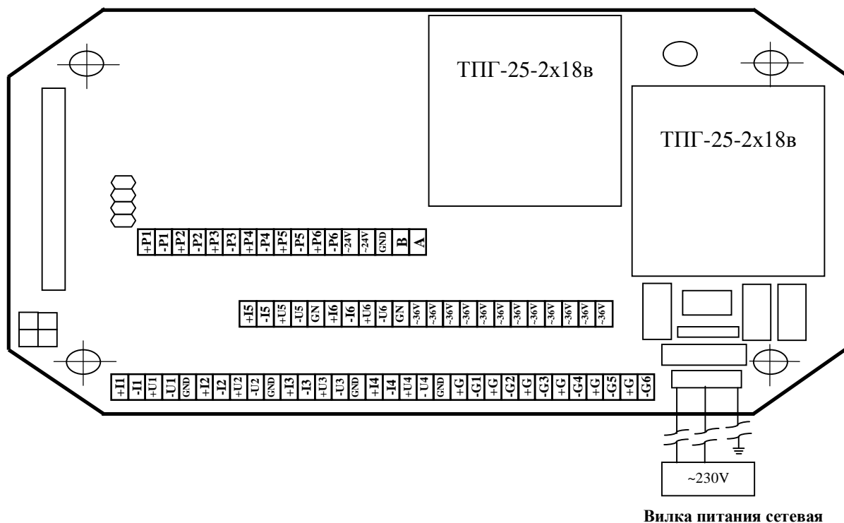
Рисунок Г.1 – Расположение элементов на клеммной плате тепловычислителя. Назначение клемм указано надписями на печатной плате.
