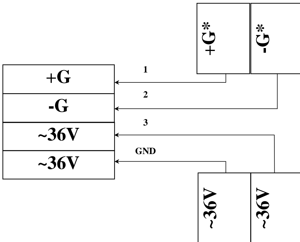
Рисунок Г.3 – Подключение датчиков потока (расходомеров) * - номер канала
