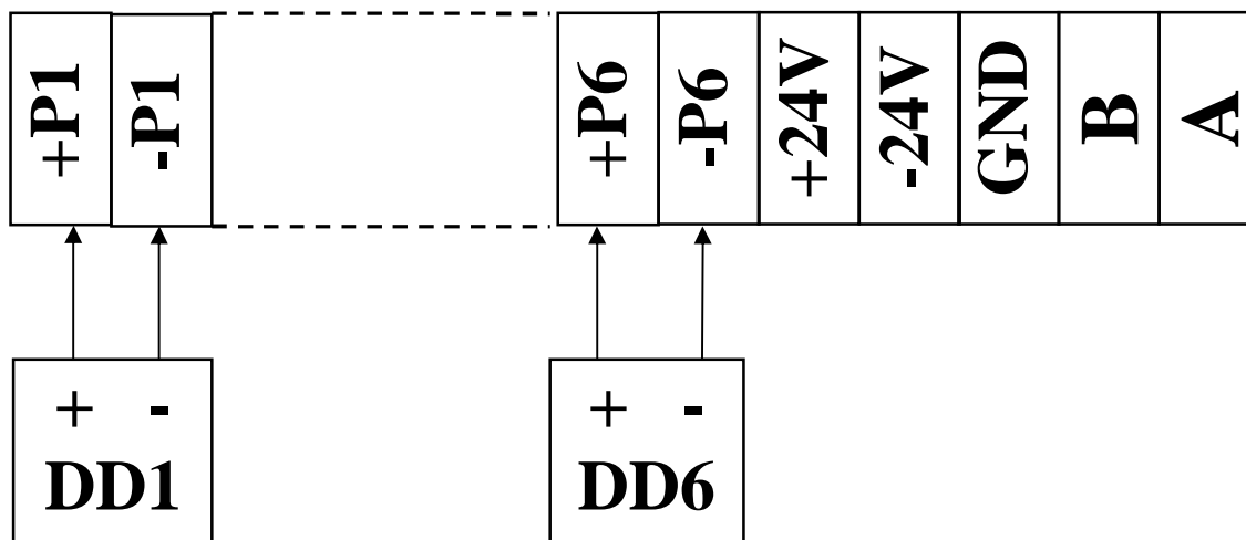
Рисунок Г.3 – Подключение датчиков потока (расходомеров) * - номер канала
